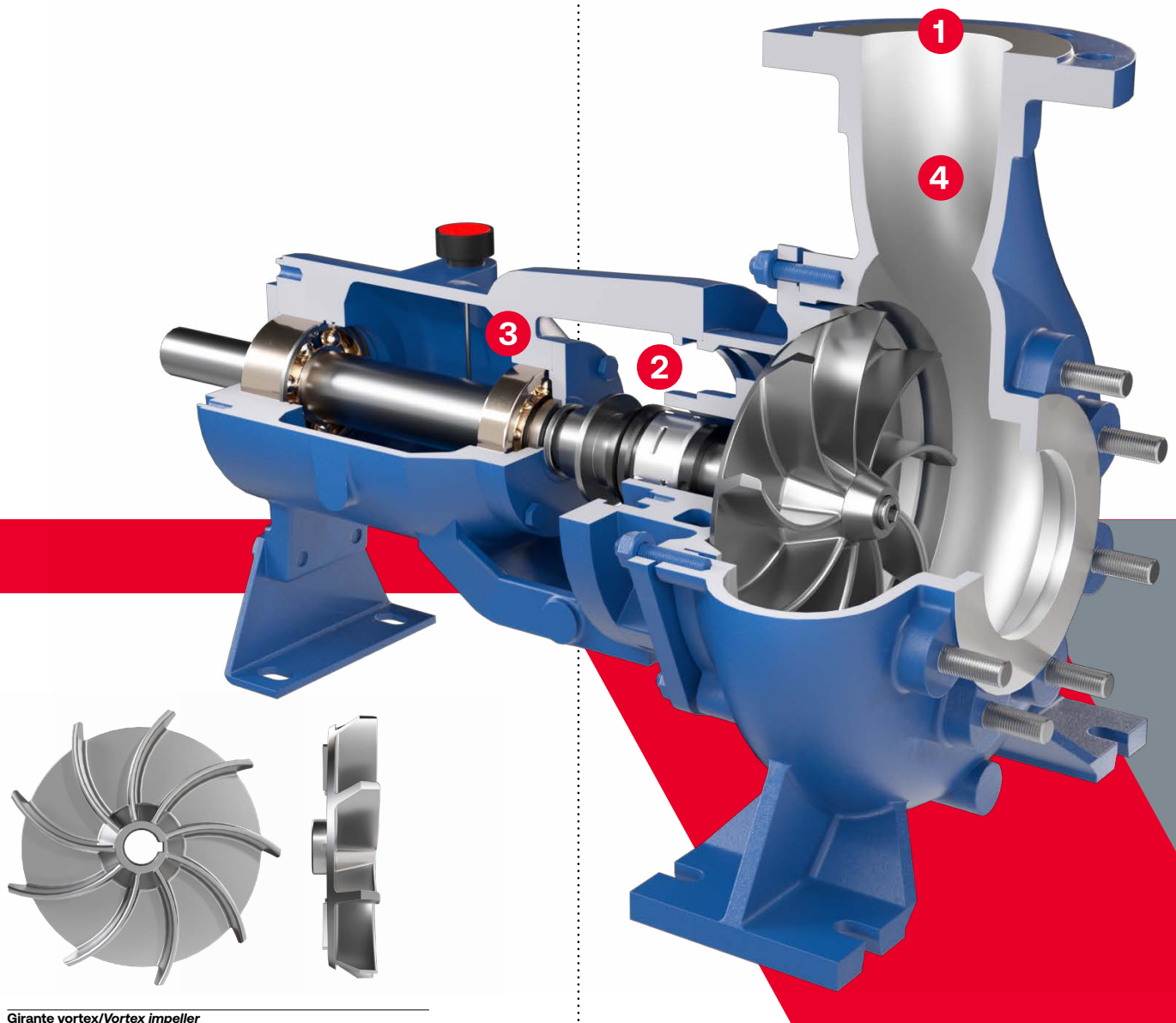
Girante vortex/Vortex impeller
