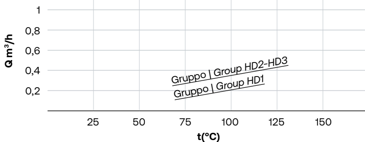
Flussaggio camera di raffreddamento esecuzione H Cooling chamber flushing H execution
