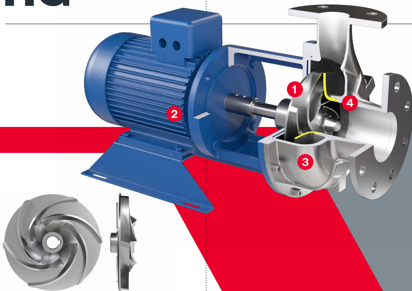
Girante aperta/Open impeller
