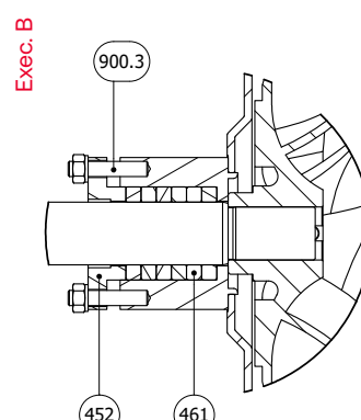
Tenuta a baderna Packing gland
