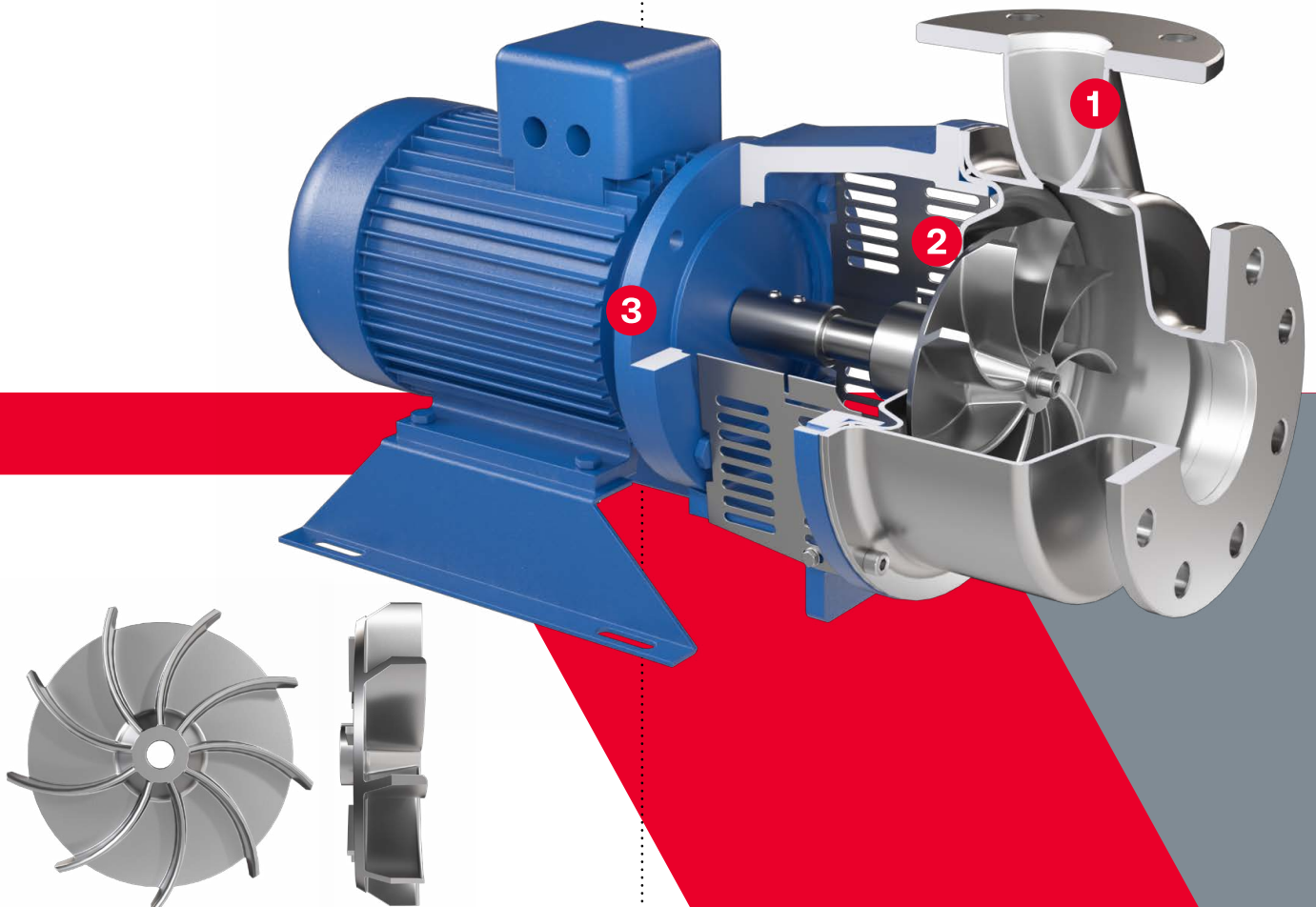
Girante vortex/Vortex impeller
